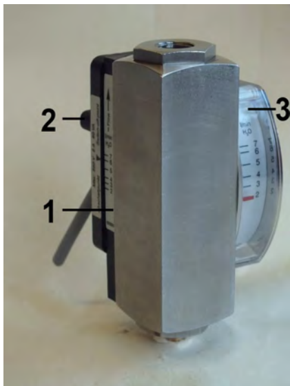
Abb. 1: Strömungswächter RVM/UA-L2 30x70
