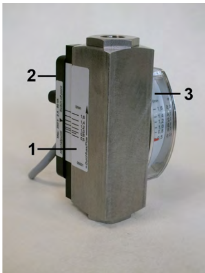
Abb. 1: Strömungswächter DKM/A-2 30x70
