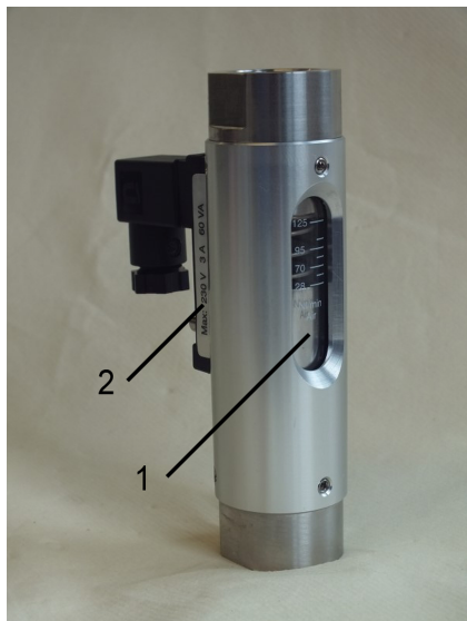
Abb. 1: Strömungswächter RVO/U-L2
