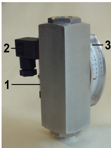
Abb. 1: Strömungswächter RVM/UA-L2
