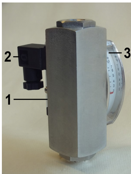
Abb. 1: Strömungswächter RVM/UA-2
