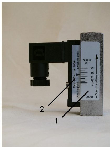
Abb. 1: Strömungswächter RVM/U-L4
