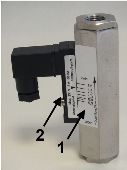
Abb. 1: Strömungswächter DKM-2
