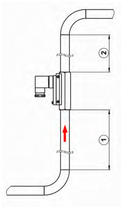
Abb. 6: Beruhigungsstrecken
