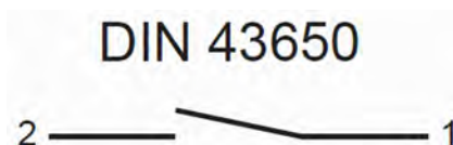
Abb. 13: Zustand des Kontaktes bei Gerät ohne Durchfluss
