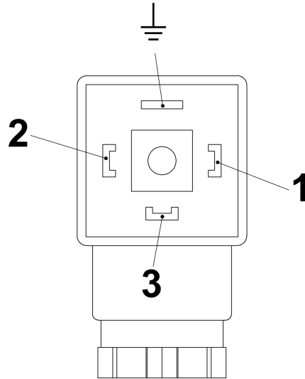
Abb. 27: Pin-Belegung Steckerdose Wechsler (Form 30x70)
