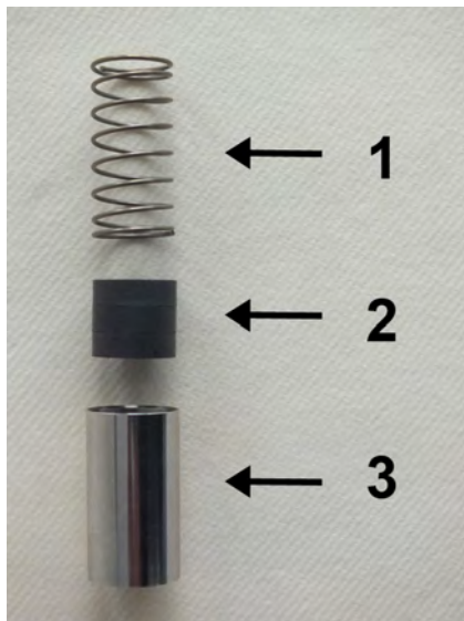
Abb. 49: Innenteile
