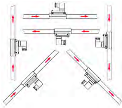
Abb. 5: Einbauposition/Durchflussrichtung
