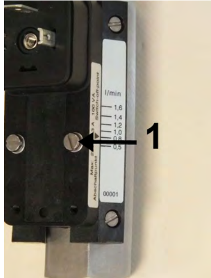
Abb. 34: Feststellschrauben lösen
