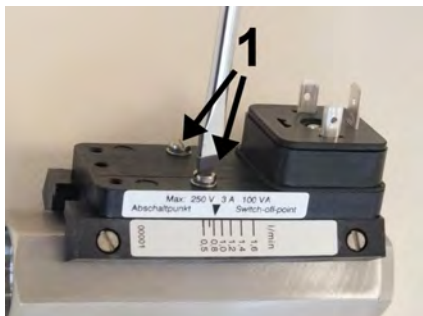
Abb. 58: Feststellschrauben lösen
