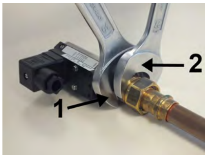
Abb. 11: Gerät einschrauben
