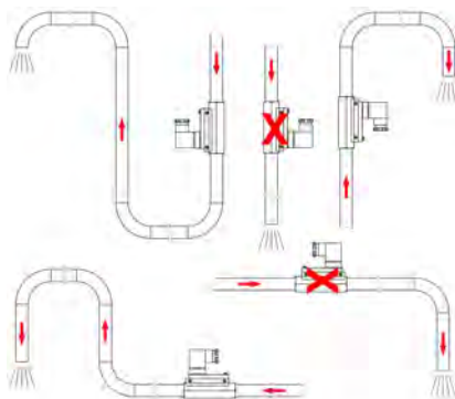
Abb. 7: Freier Auslauf
