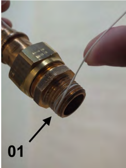
Abb. 9: Dichtfaden aufbringen
