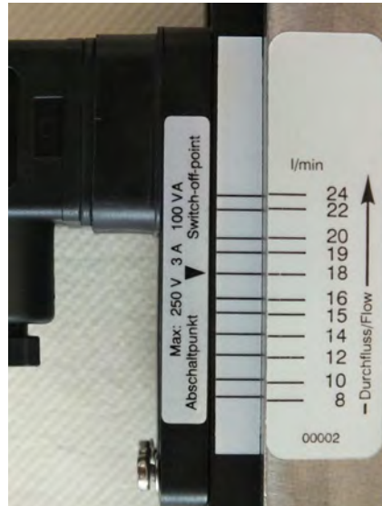
Abb. 4: Körperskala (Beispiel)
