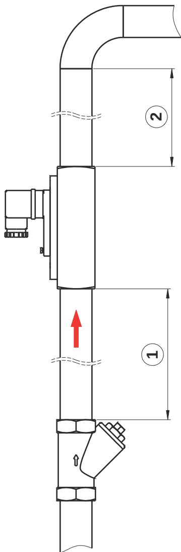
Abb. 8: Schmutzfänger
