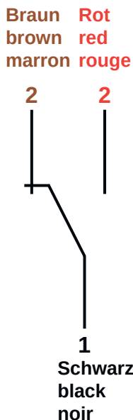
Abb. 21: Zustand des Kontakts bei Gerät ohne Durchfluss
