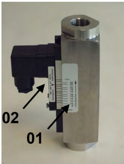
Abb. 1: Strömungswächter RVM/U-1
