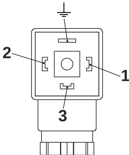
Abb. 16: Pin-Belegung Steckerdose Wechsler (Erde-Anschluss nicht genutzt)
