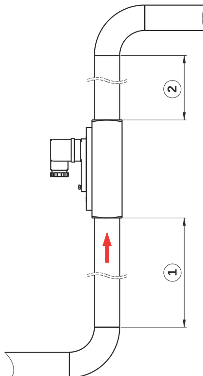
Abb. 6: Beruhigungsstrecken
