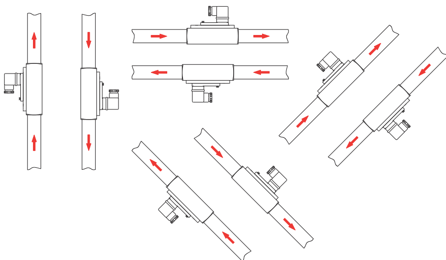
Abb. 5: Einbauposition/Durchflussrichtung
