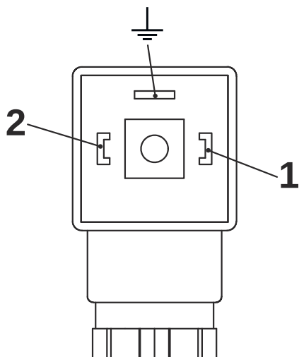
Abb. 14: Pin-Belegung Steckerdose Schließer (Erde-Anschluss nicht genutzt)
