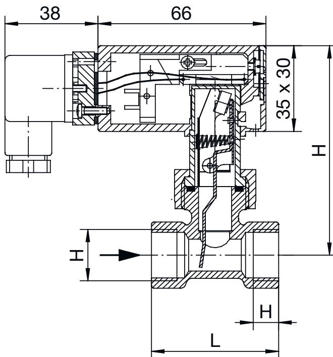
Abb. 6: Maßblatt
