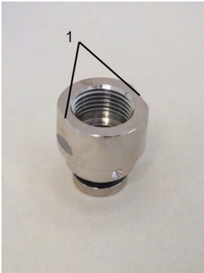
Fig. 44: Spanner flats
