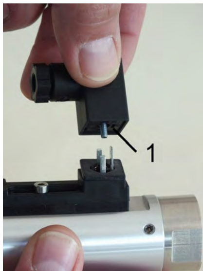
Fig. 21: Remove socket
