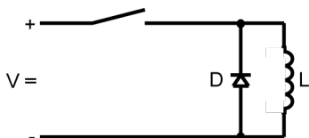
Abb. 28: Beispiel 1
