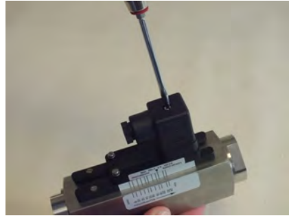
Abb. 61: Steckerdose lösen
