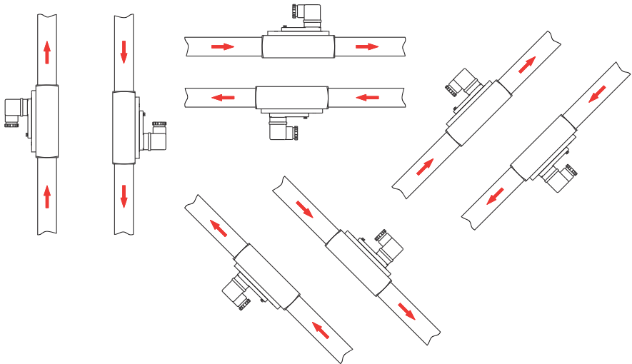
Abb. 5: Einbauposition/Durchflussrichtung
