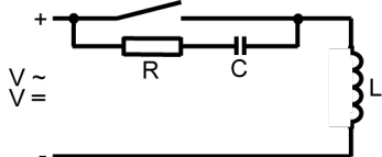
Abb. 29: Beispiel 2
