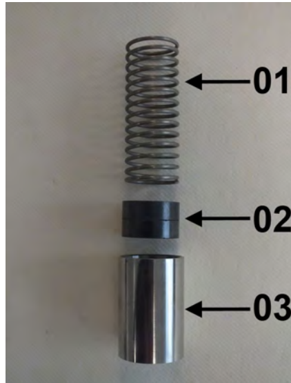
Abb. 42: Feder, Magnete und Schwebekörper
