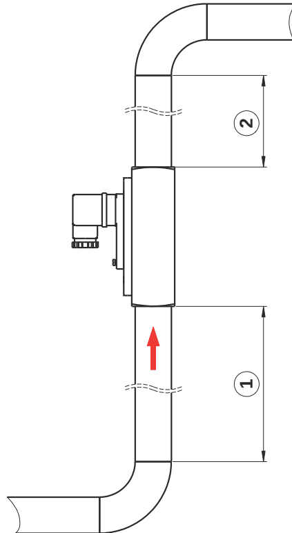
Abb. 6: Beruhigungsstrecken
