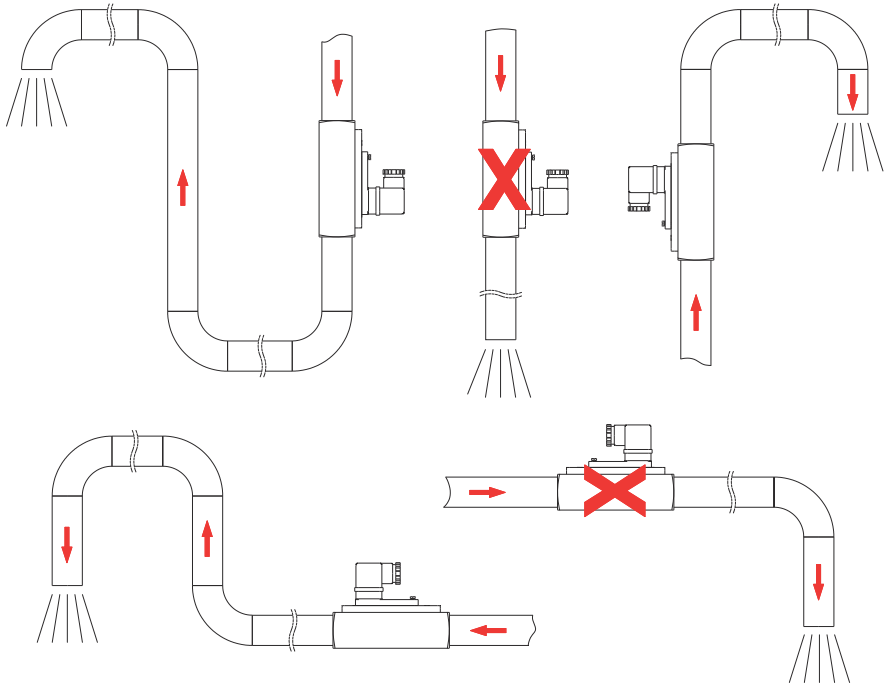
Abb. 7: Freier Auslauf
