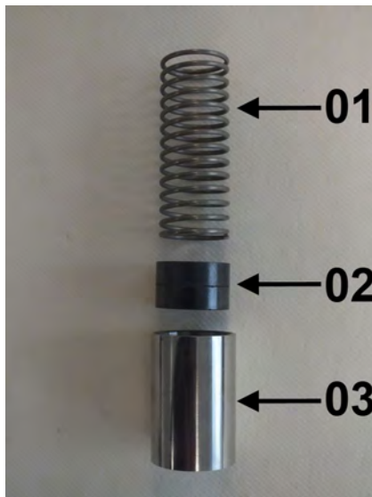
Abb. 54: Innenteile
