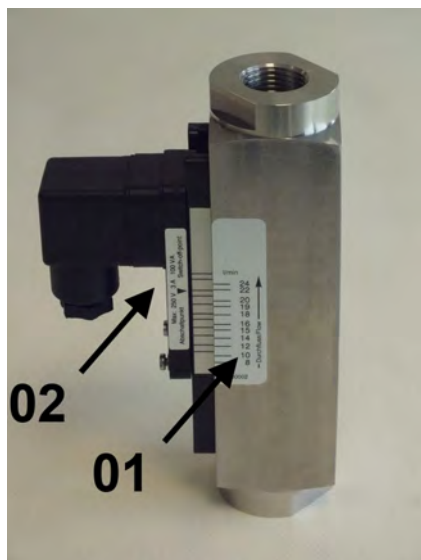
Abb. 1: Strömungswächter DKM-1
