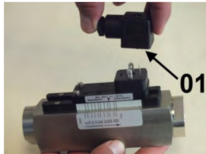
Abb. 62: Steckerdose abziehen
