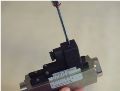
Abb. 22: Steckerdose lösen
