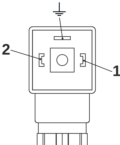
Abb. 13: Pin-Belegung Steckerdose Schließer (Erde-Anschluss nicht genutzt)
