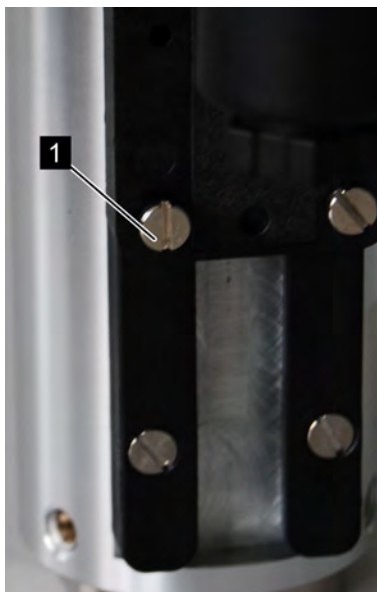
Abb. 32: Feststellschrauben lösen
