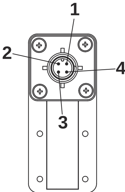
Abb. 16: Pin-Belegung Gerätestecker M12x1 (Form 30x70)
