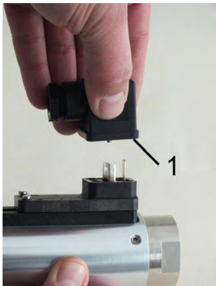
Abb. 54: Steckerdose abziehen
