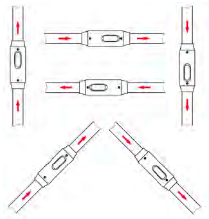
Abb. 5: Einbauposition/Durchflussrichtung
