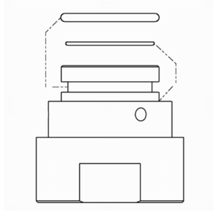
Abb. 42: Position der O-Ringe
