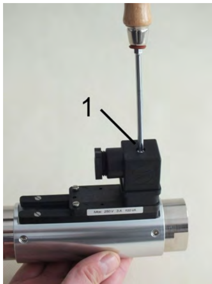
Abb. 53: Steckerdose lösen
