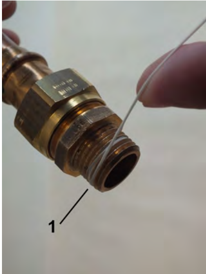
Abb. 8: Dichtfaden aufbringen
