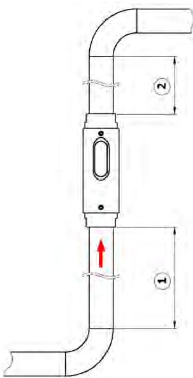
Abb. 6: Beruhigungsstrecken
