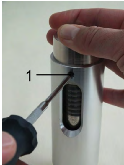
Abb. 51: Innensechskantschrauben anziehen
