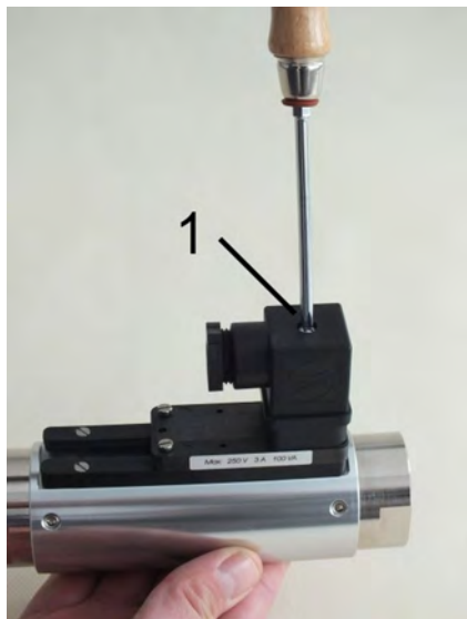
Abb. 21: Steckerdose lösen
