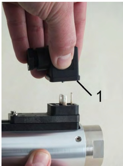
Abb. 22: Steckerdose abziehen
