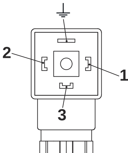
Abb. 15: Pin-Belegung Steckerdose Wechsler (Erde-Anschluss nicht genutzt)
