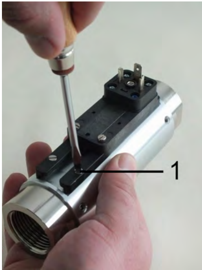
Abb. 56: Führungsleiste lösen
