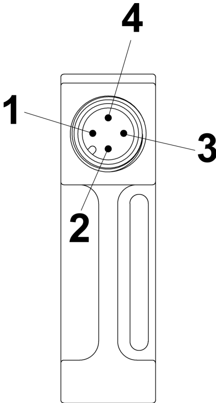
Abb. 18: Pin-Belegung Gerätestecker M12x1 (Form 15x50)
