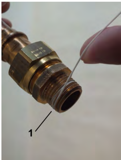
Abb. 10: Dichtfaden aufbringen
