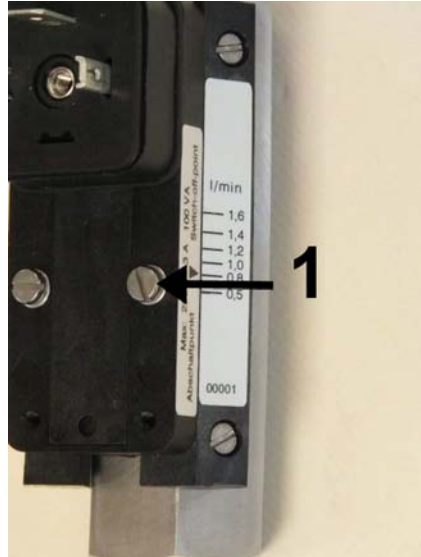
Abb. 31: Feststellschrauben lösen
