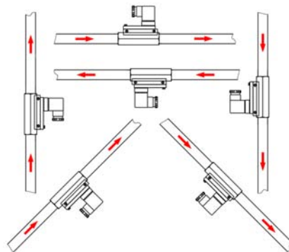
Abb. 5: Einbauposition/Durchflussrichtung
