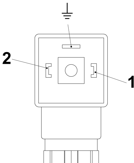
Abb. 23: Pin-Belegung Steckerdose Schließer (Form 30x70)
