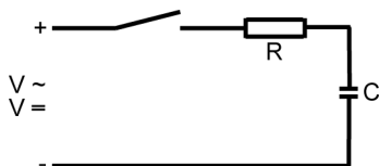
Abb. 27: Schutzmaßnahme bei kapazitiver Belastung
