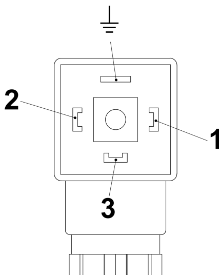
Abb. 24: Pin-Belegung Steckerdose Wechsler (Form 30x70)
