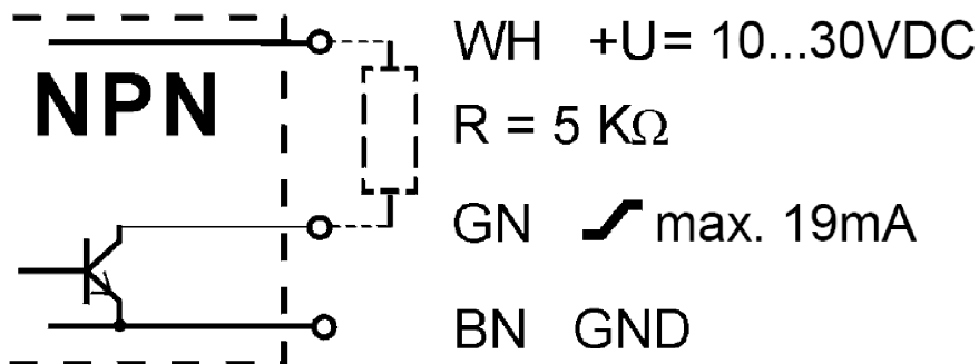
Abb. 3: Anschlussbild
