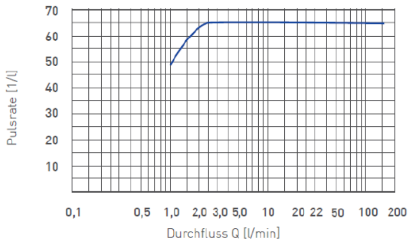
Abb. 8: Impulskennlinie
