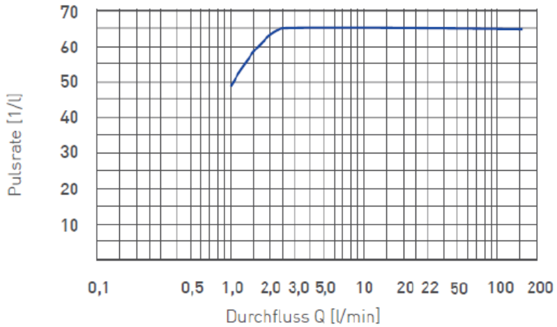
Abb. 4: Impulskennlinie
