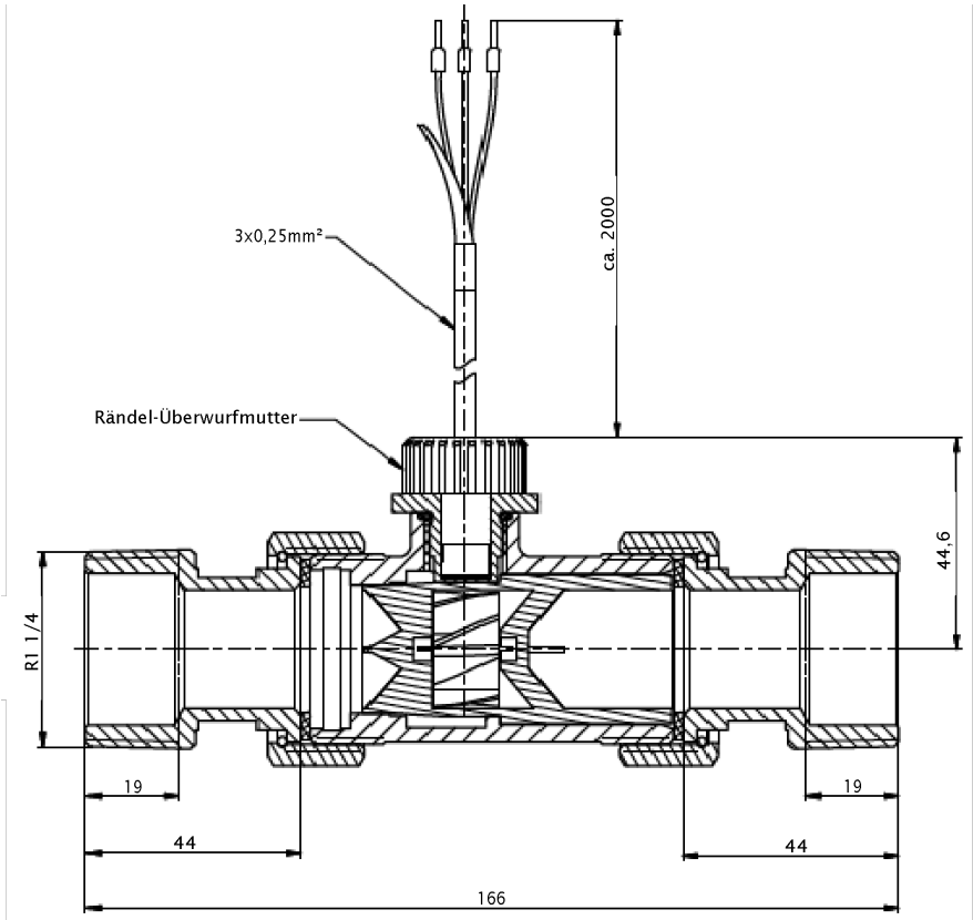
Abb. 7: Maßblatt
