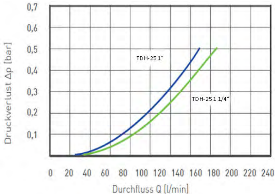
Abb. 9: Druckverlust
