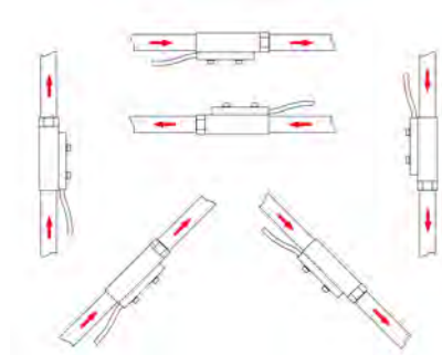
Abb. 5: Einbauposition/Durchflussrichtung
