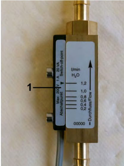
Abb. 3: Schaltkontakt mit Anschlusskabel
