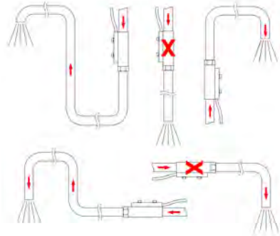
Abb. 7: Freier Auslauf
