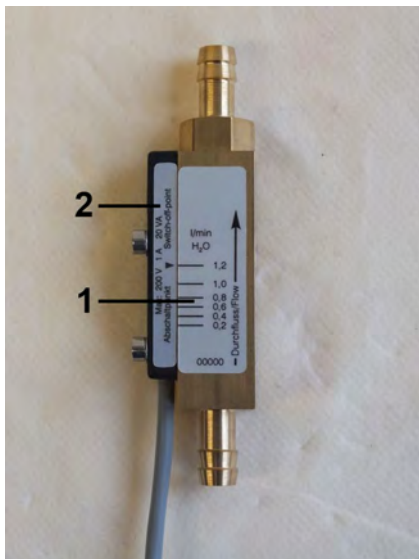
Abb. 1: Strömungswächter RVM/U-S4
